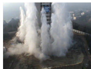
Déconstruction à Rilleux la Pape (69) par foudroyage avec pulvérisation pyrotechnique de rideaux d'eaux anti poussières.
