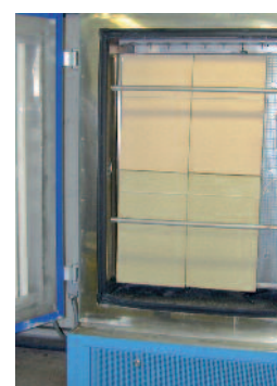
Essai sur système ITE dans une enceinte climatique
